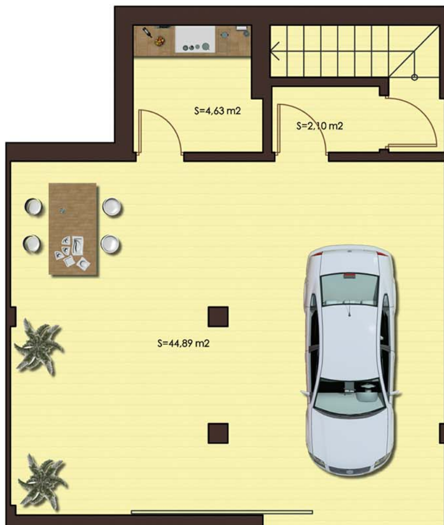
Planta Sotano tipo 2. Sc:63,41m 2
